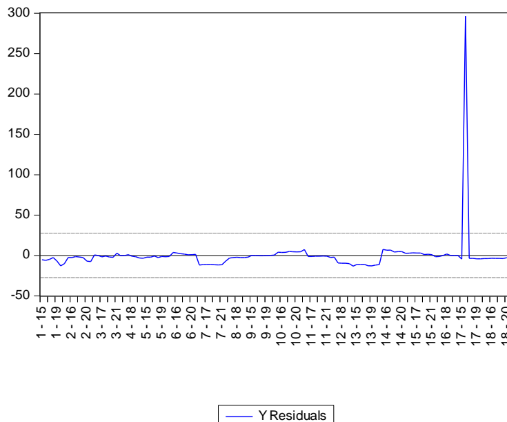
Gambar 2. Hasil Uji Heteroskedastisitas Model Regresi Data Panel Random Effect Negara Kawasan Asia Sumber: EViews 10
